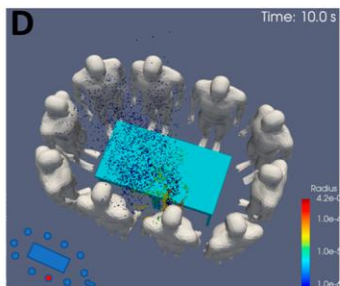
マスク無・ソーシャルディスタンスを取らずに屋外で咳をした時の実験
