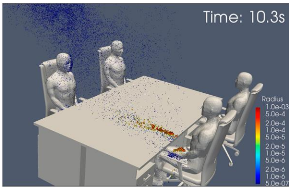
出典：神戸大学 富岳スーパーコンピューターによるシミュレーション
